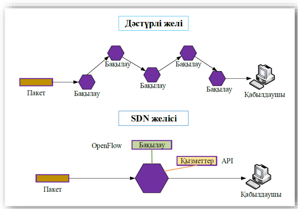
Сурет 2. Дәстүрлі желіде және SDN желісінде пакеттерді жіберу
