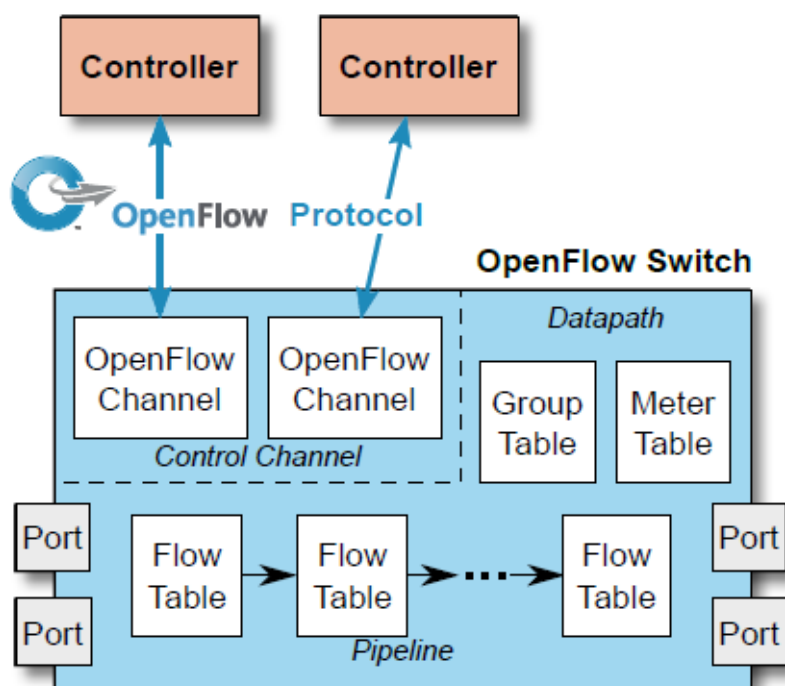
Сурет 3. OpenFlow маршрутизаторының құрылымы
