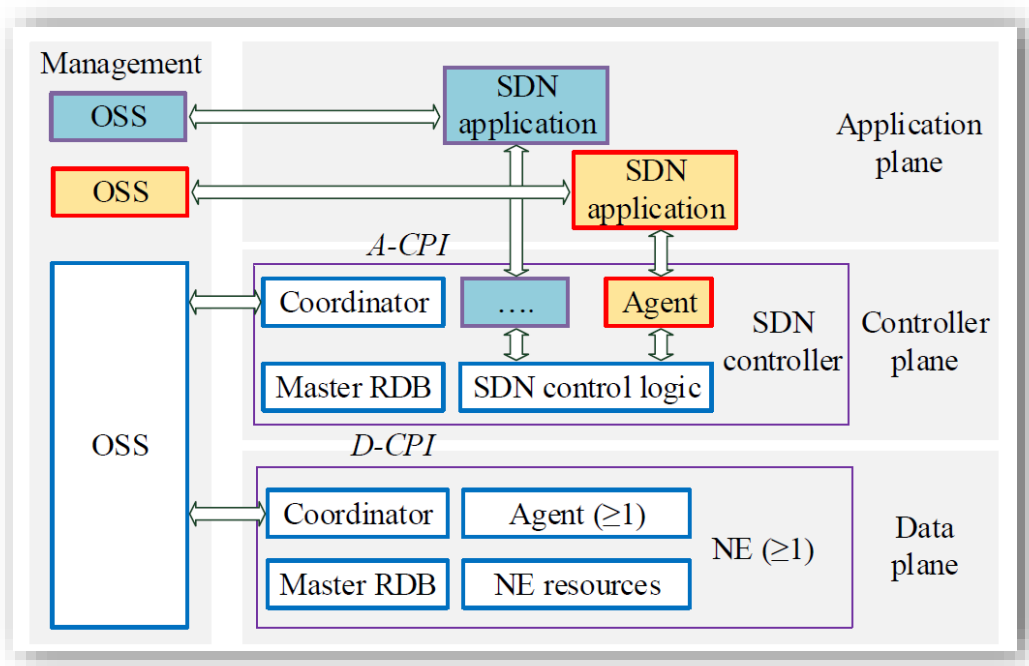
Сурет 1. SDN архитектурасы
